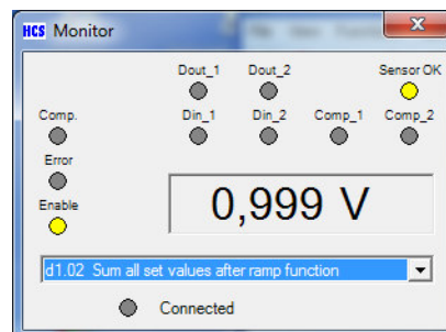
Figure 38: ODC Enabled, digital value set.
